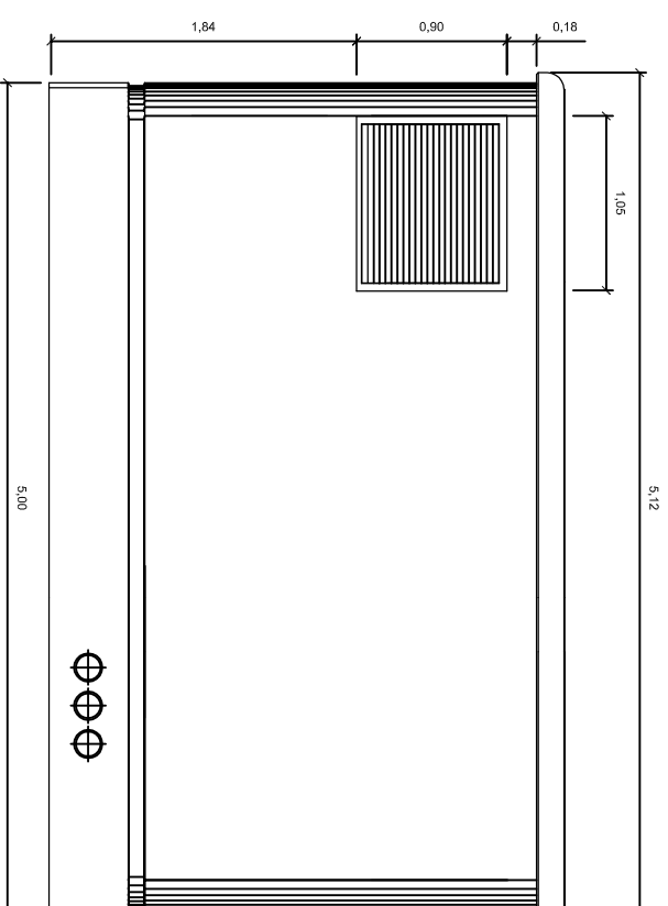
ALÇADO POSTERIOR
