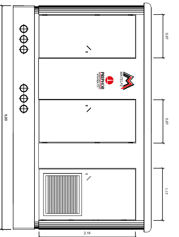
ALÇADO PRINCIPAL
