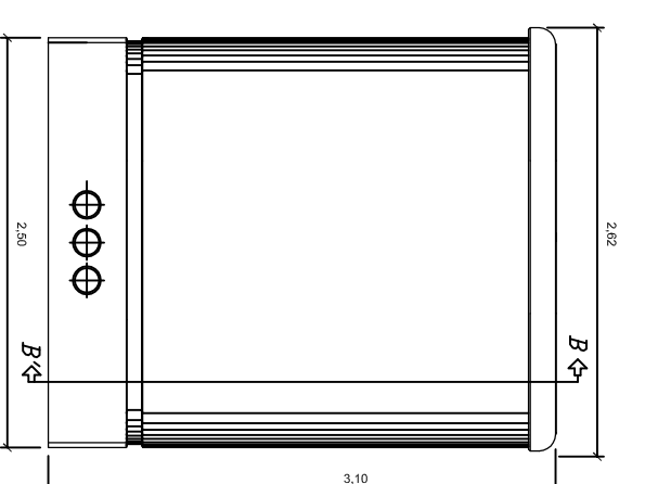
ALÇADO LATERAL ESQUERDA
